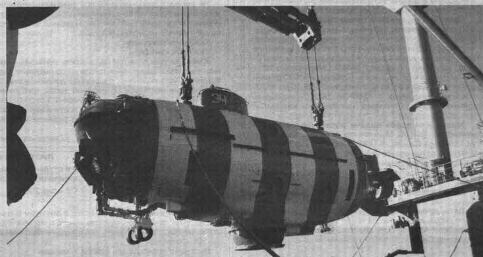
Выгрузка АС-34 из трюма спасательного судна «Георгий Титов».
